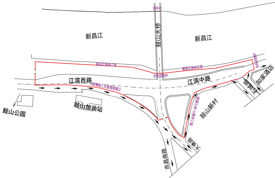
江滨西路与鼓山大桥节点改造工程封道范围示意图
