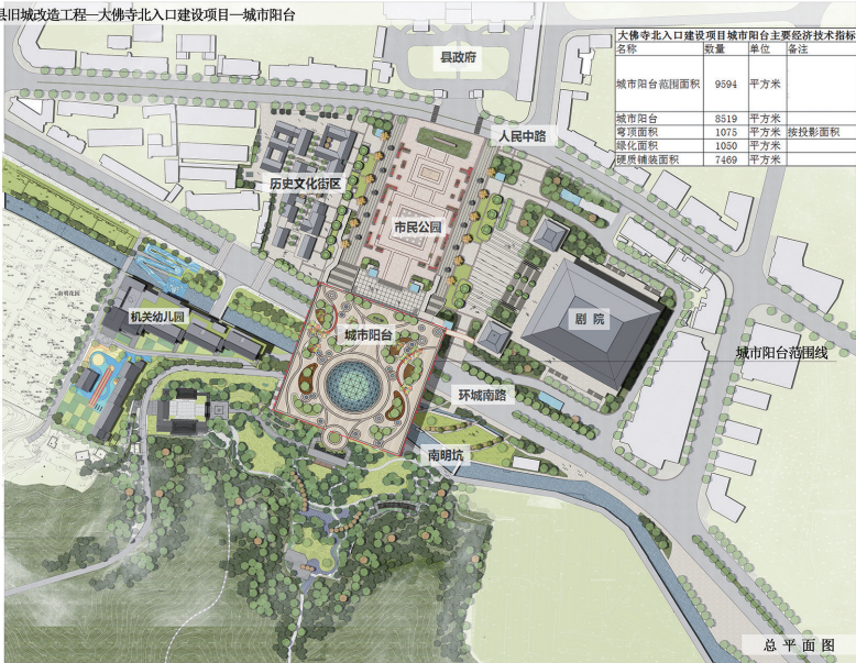
总平面图
