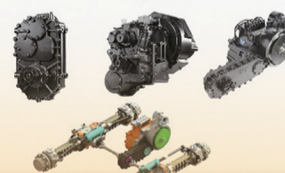
3.5-5T伸缩臂叉车传动系统
