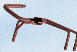
叶轮式分配器组件
