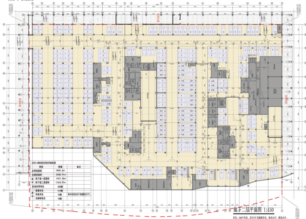
地下二层平面图 Basement Level 2 Floor Plan
